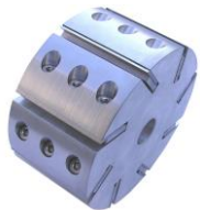
82W 平型カッターボデー 部品番号 H82WB 寸法 82Wxφ160
