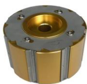
100W 平型カッターボデー 部品番号 HE100WB 寸法 100xφ160
